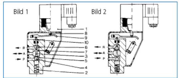
Elektromagnet spannungslos
